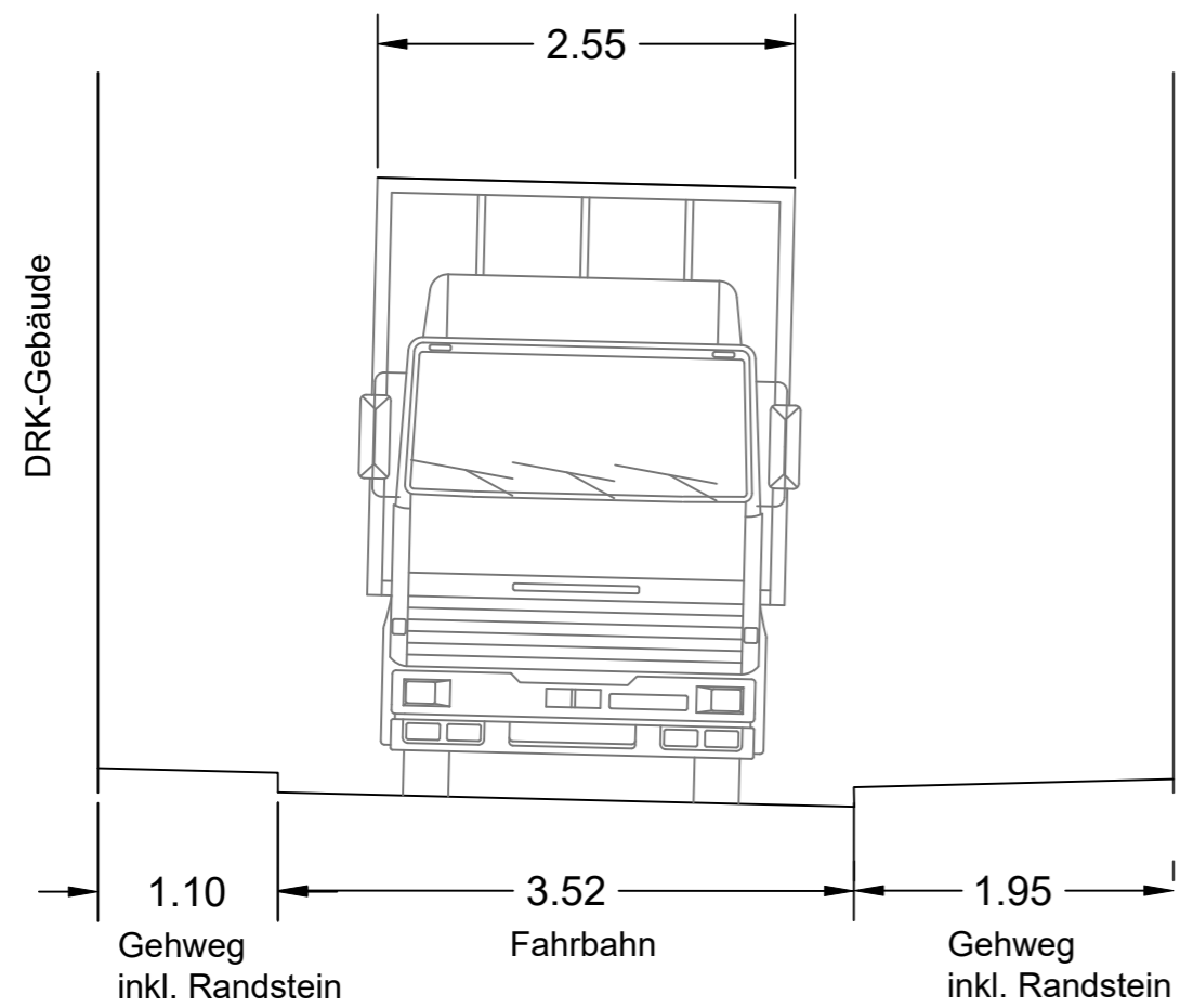
Schleppkurve 3-achsiges Müllfahrzeug
